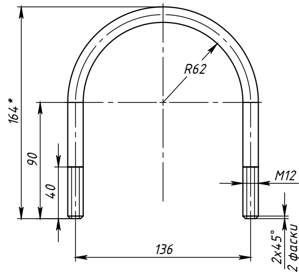
Поз.5 (Хомут)
