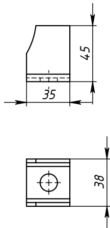
Поз.4 (Ушко)
