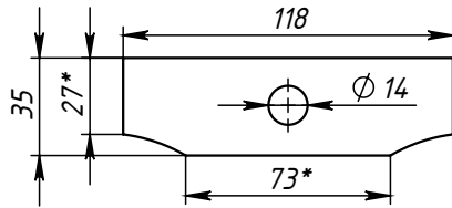
Поз.4 (Ушко) развертка
