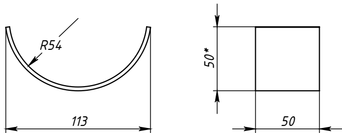
Поз.3 (Ложемент)
